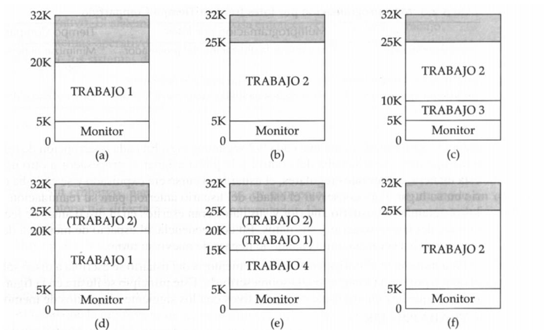
FIGURA 2.9 Funcionamiento del CTSS
