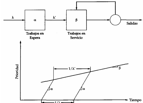
FIGURA 8.19 Round-robin egoísta
