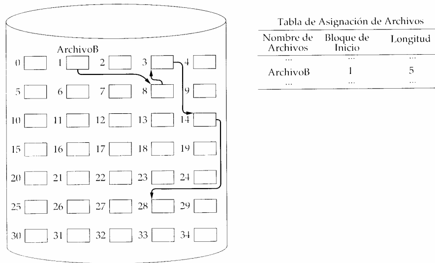
FIGURA 11.9 Asignación encadenada
