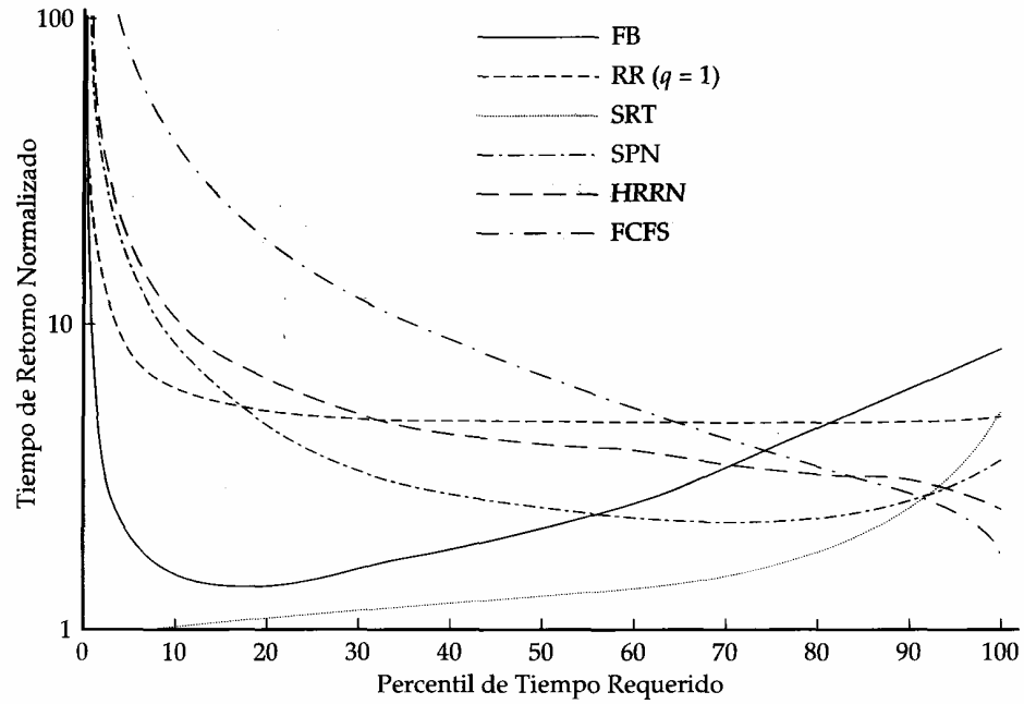
FIGURA 8.15 Resultados de la simulación para el tiempo de retorno normalizado
