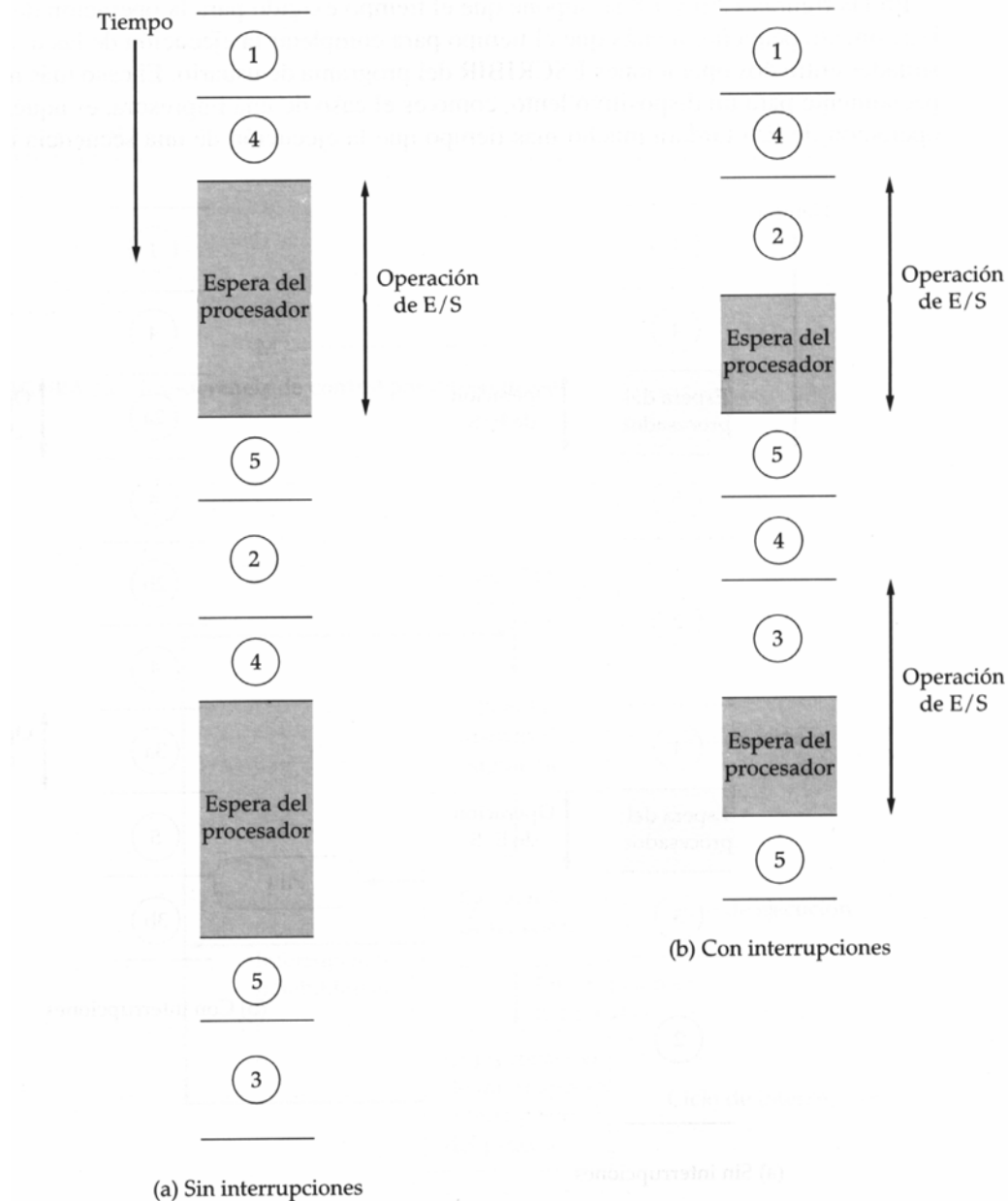
Figura 1.9 Diagramas de tiempo de un programa; espera larga de E/S
