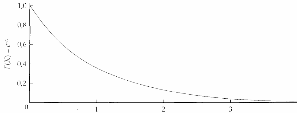
(b) Função de densidade de probabilidade exponencial
