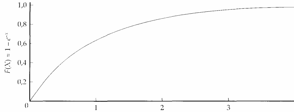
(a) Função de distribuição de probabilidade exponencial
