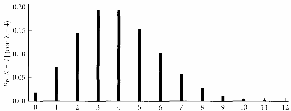
(c) Distribuição de probabilidade de Poisson
