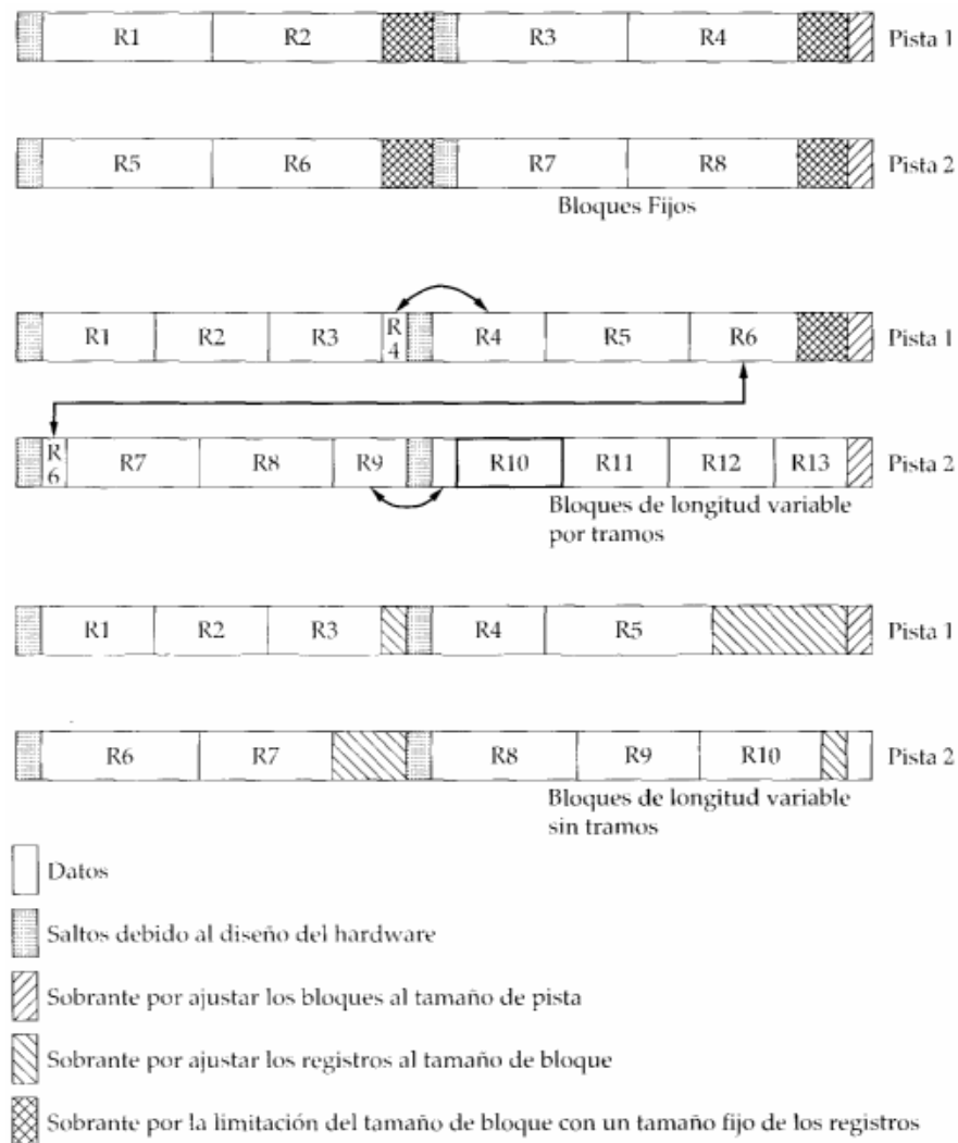
FIGURA 11.6 Métodos de agrupación de registros [WIED87]
